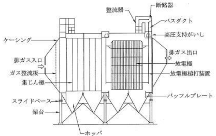
図 3-2 電気集じん器の例
